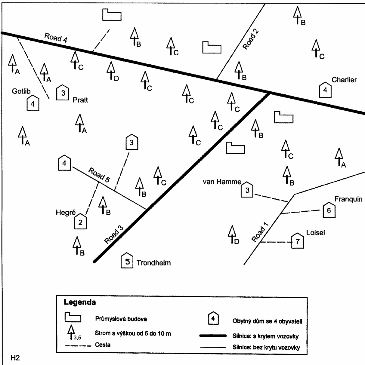
Obrázek G.3 – Grafická reprezentace „univerza diskurzu“
