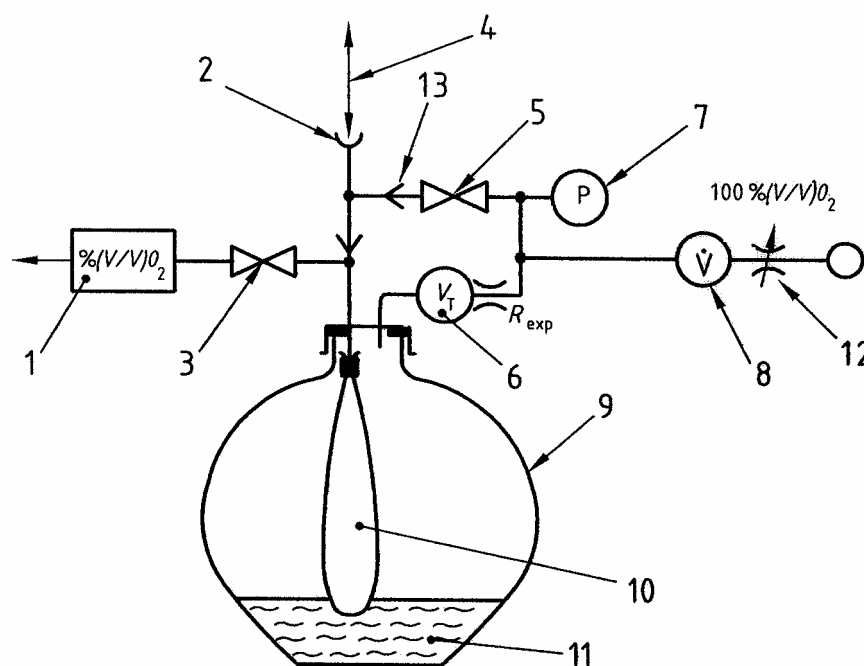
Obrázek A.3 b) – Zkušební zařízení
