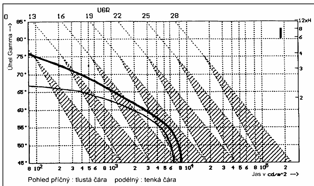
Diagram I pro případy typického jasu pozadí s čarami jasu daného svítidla
