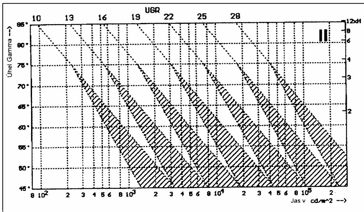
Diagram II pro případy relativně vysokého jasu pozadí
