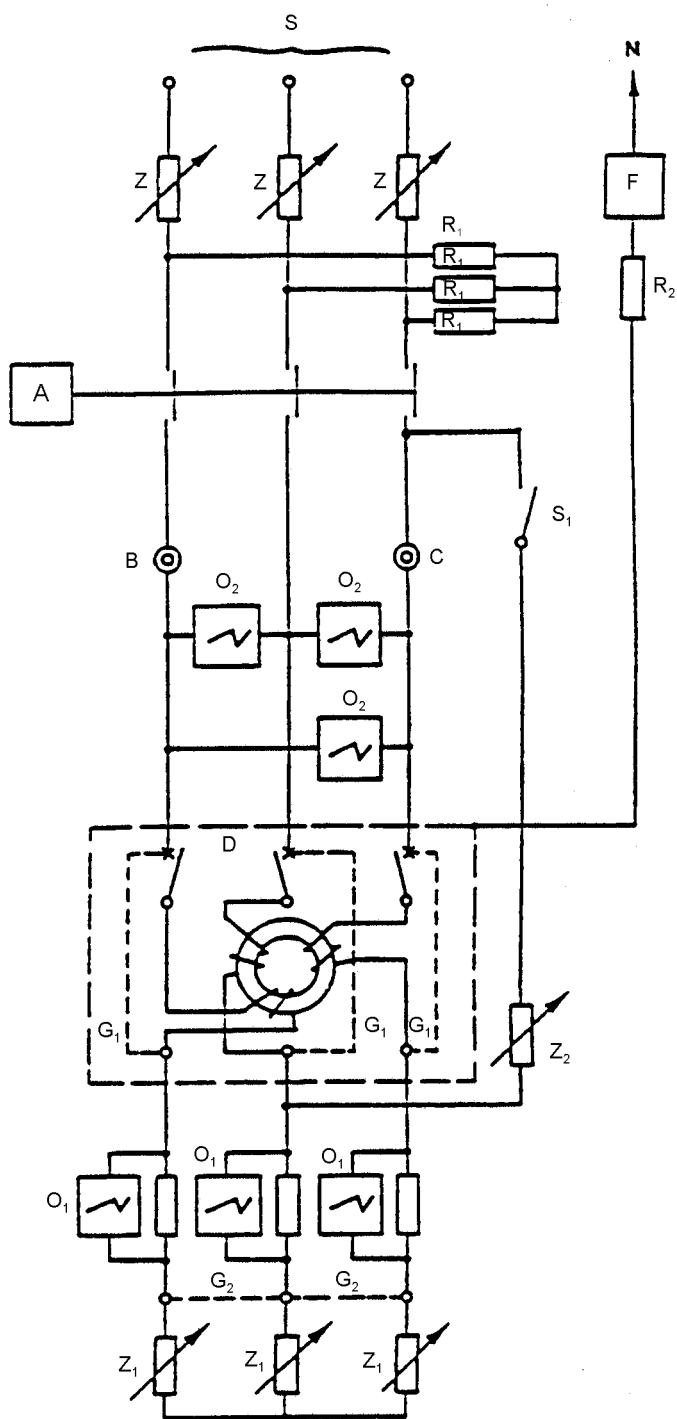
Obrázek Z2 – Zkušební obvod pro ověření jmenovité zkratové schopnosti trojpolového RCBO v případě trojfázového obvodu (9.12)
