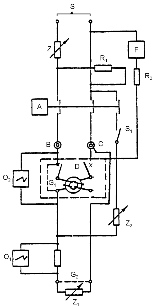
Obrázek Z1 – Zkušební obvod pro zkoušku při snížených zkratových proudech a pro ověření jmenovité reziduální zapínací a vypínací schopnosti ( I_{\Delta m} ) RCBO
