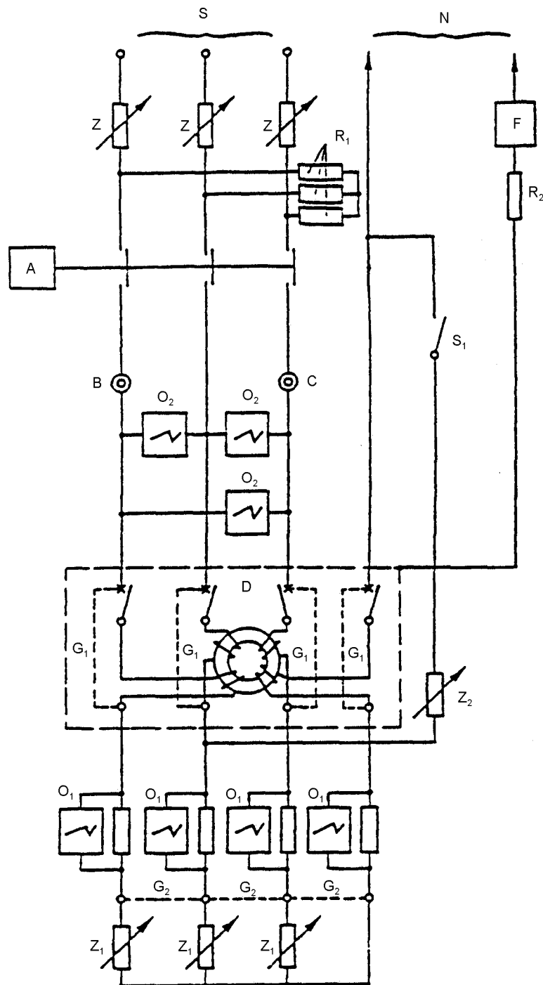
Obrázek Z3 – Zkušební obvod pro ověření jmenovité zkratové schopnosti čtyřpólového RCBO v případě trojfázového obvodu se středním vodičem (9.12)
