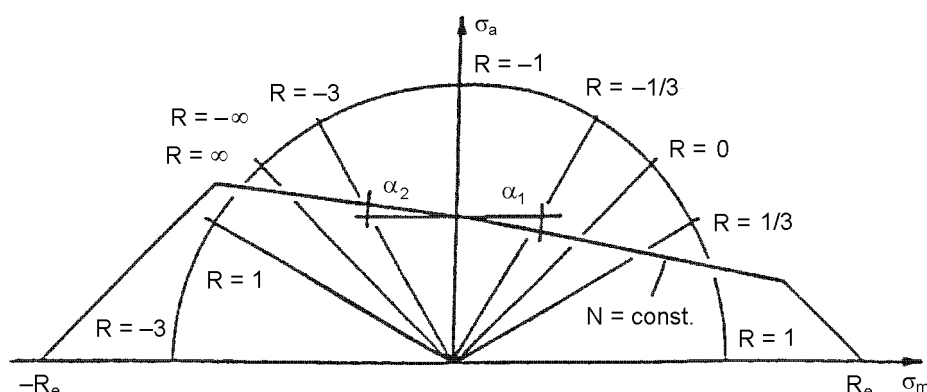
Obrázek 7 – Rovina \sigma_a - \sigma_m pro uvažovaný prvek při prokázání únavové pevnosti (zjednodušený Haighův diagram)
