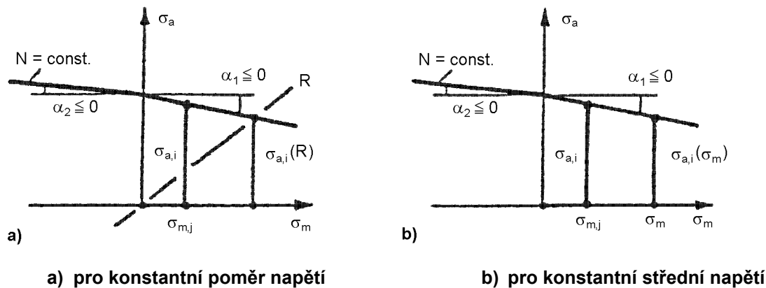
Obrázek 8 – Transformace cyklů napětí
