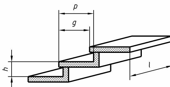
Obrázek 3 – Rozměrové parametry pro schodiště a žebříková schodiště
