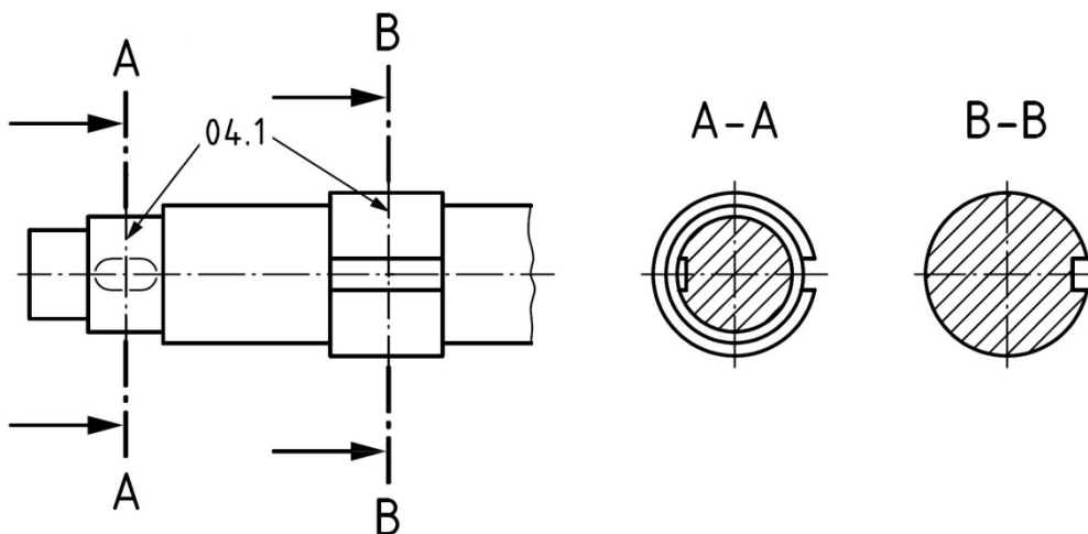
Obrázek NA.1.1 – Použití čáry č. 04.1.6
