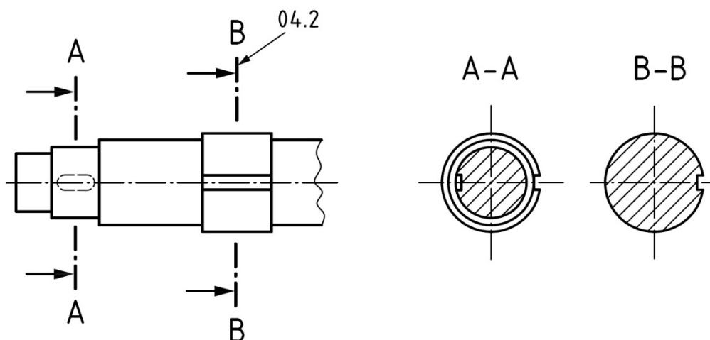
Obrázek NA.1.2 – Použití čáry č. 04.2.2
